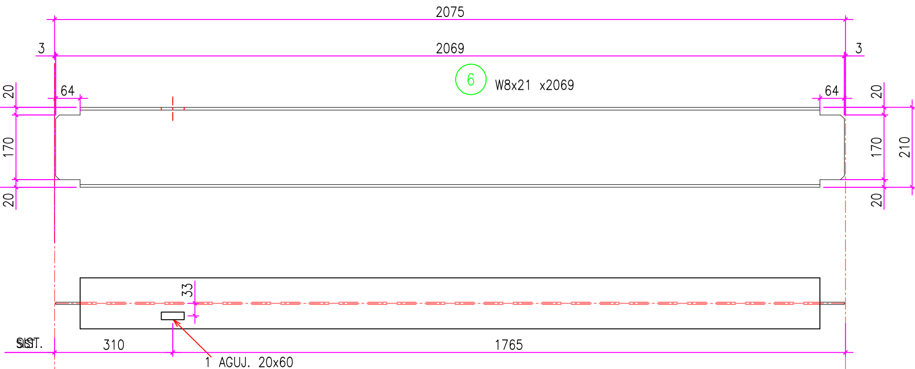
VIGA V8 CANT.: 1 ESC.: 1:10
