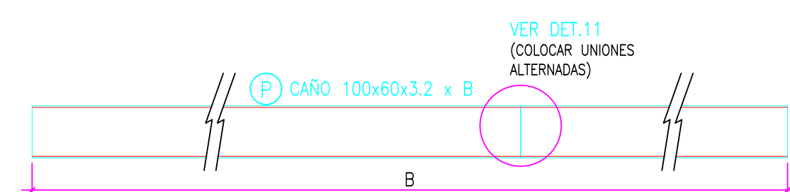
CORREAS TECHO ESCALA 1:10
