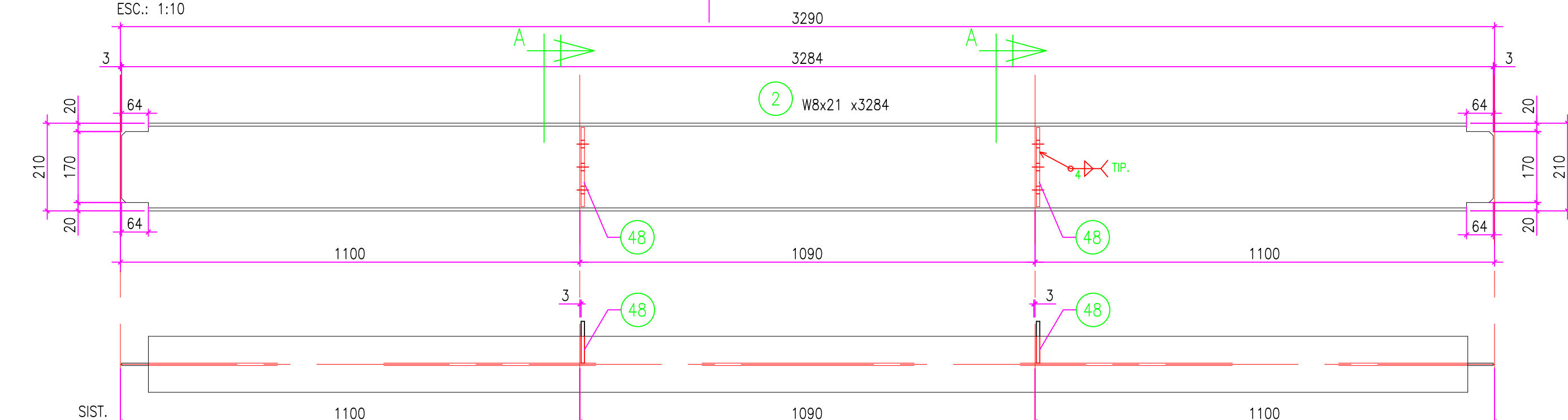
VIGA V12 CANT.: 1 (S/ DIBUJO) VIGA V18 CANT.: 1 (MANO OPUESTA) ESC.: 1:10
