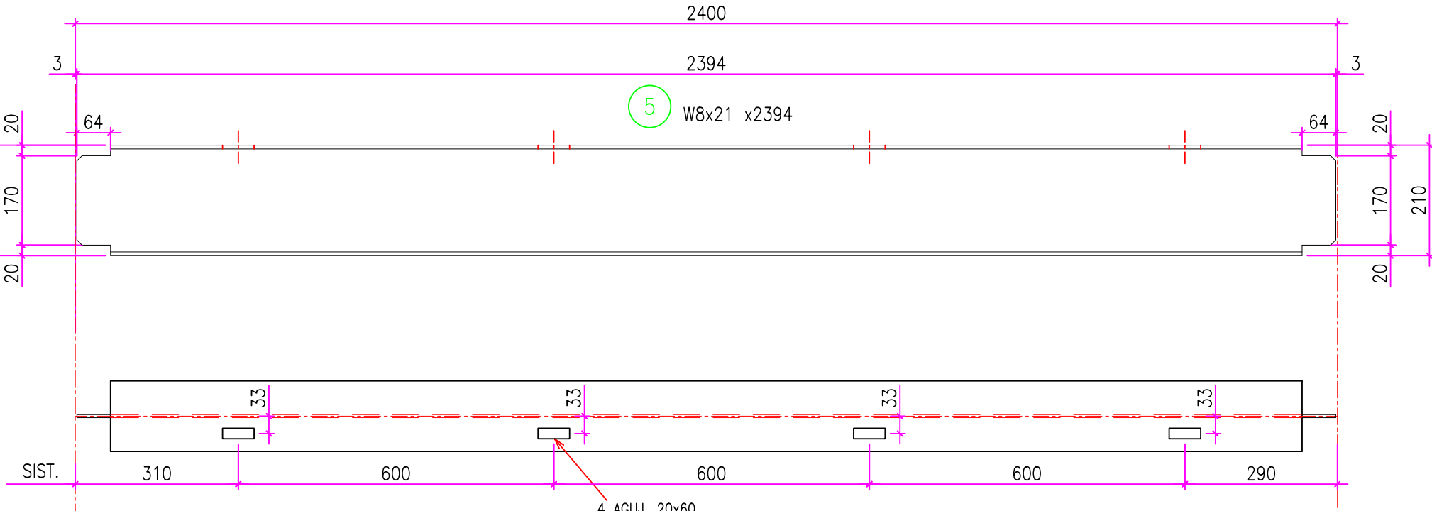
VIGA V7 CANT.: 1 ESC.: 1:10
