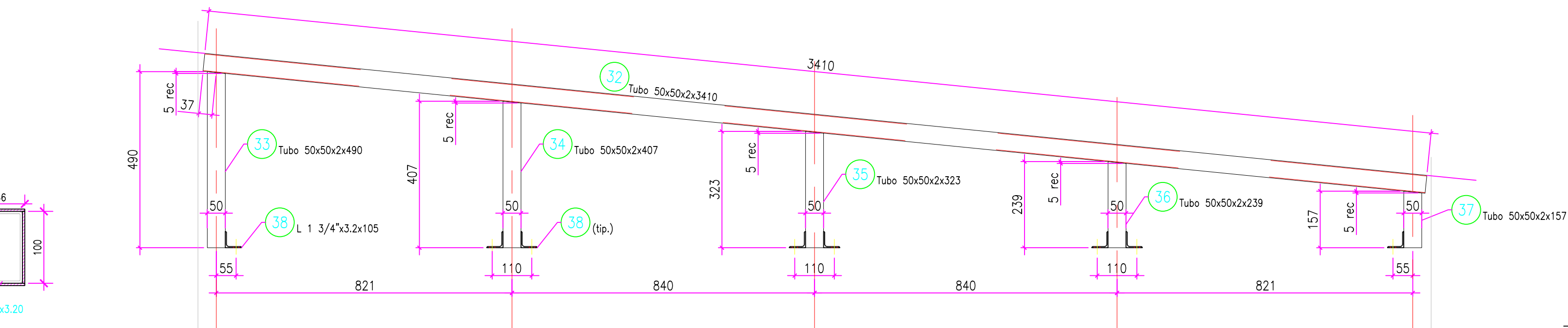
DET. SOPORTE TECHO SPT-01 (CANT.13) ESC. 1:10
