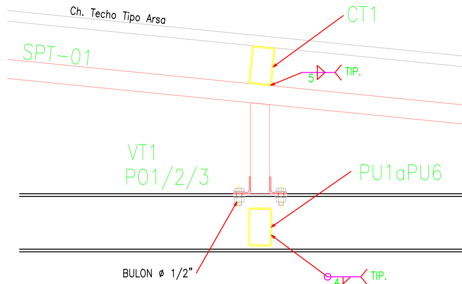
DET. 6 ESCALA 1:10
