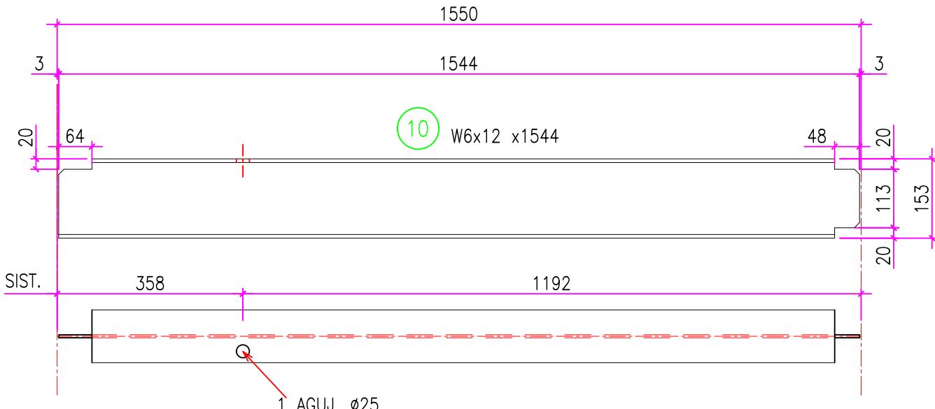
VIGA V3 CANT.: 3 ESC.: 1:10
