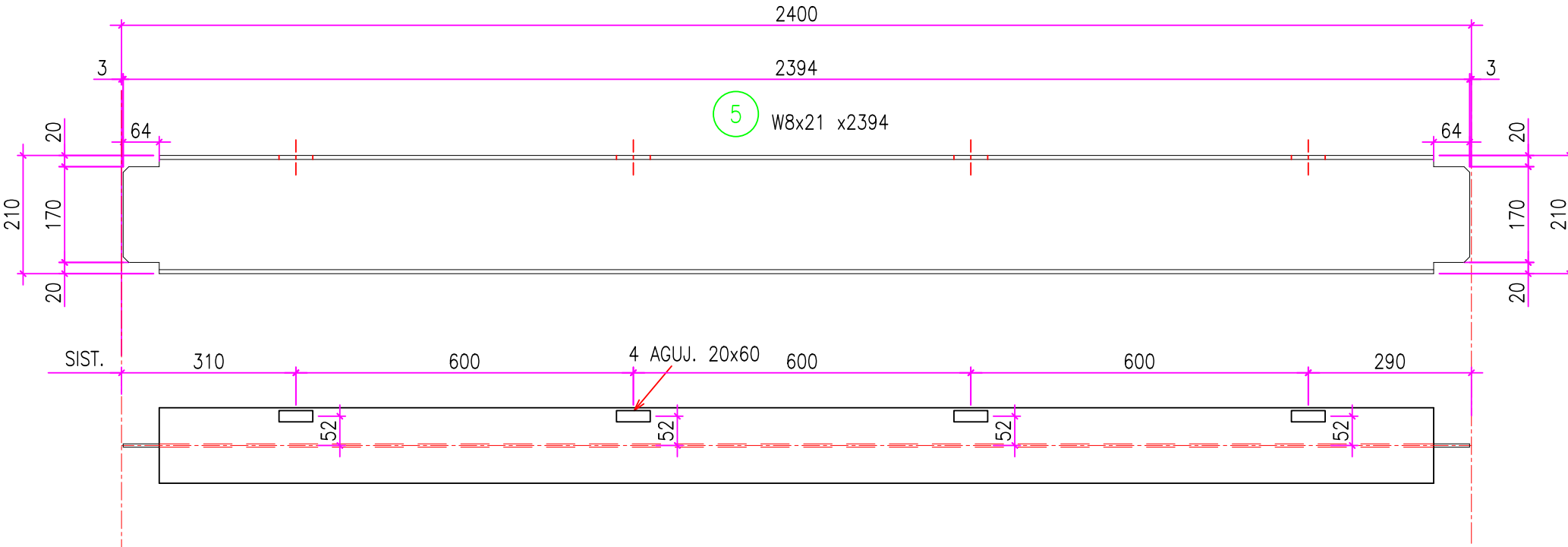
VIGA V10 CANT.: 1 ESC.: 1:10
