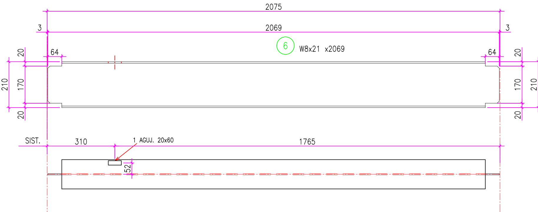
VIGA V11 CANT.: 1 ESC.: 1:10
