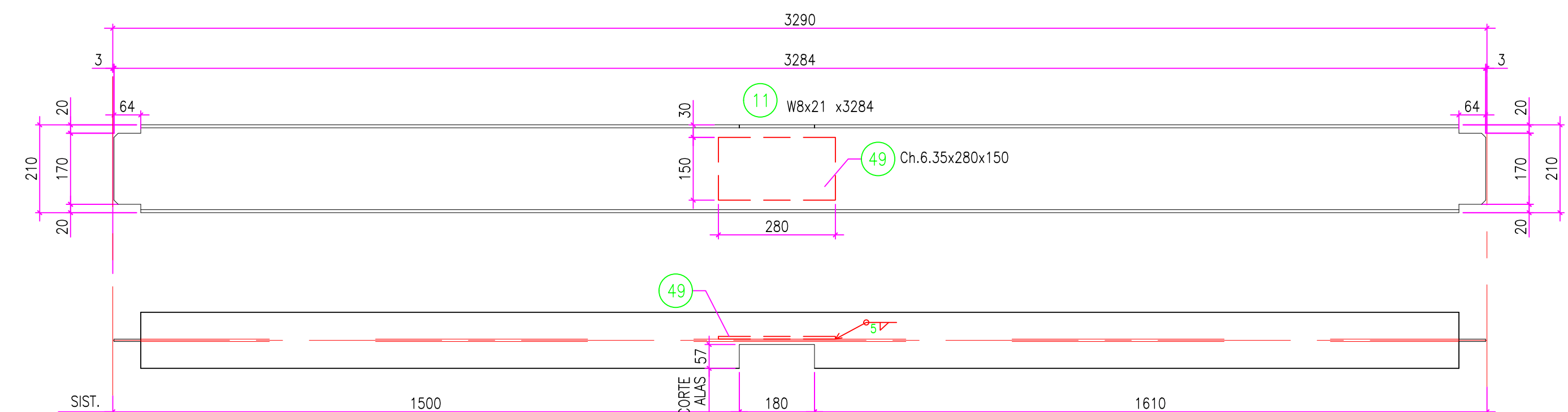
VIGA V16 CANT.: 2 ESC.: 1:10
