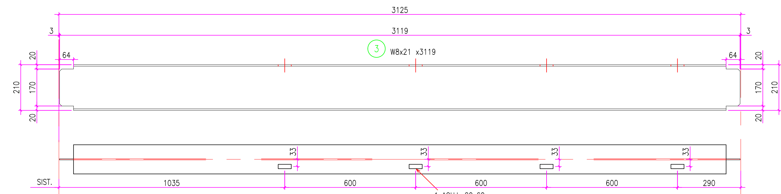
VIGA V6 CANT.: 1 ESC.: 1:10
