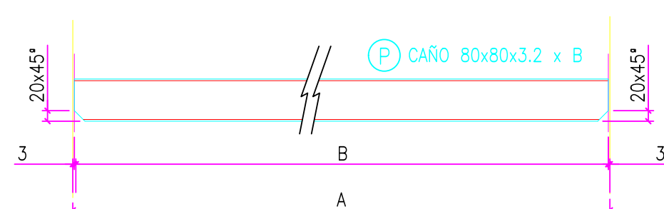
VIGA V12 CANT.: 1 (S/ DIBUJO) VIGA V18 CANT.: 1 (MANO OPUESTA) ESC.: 1:10
