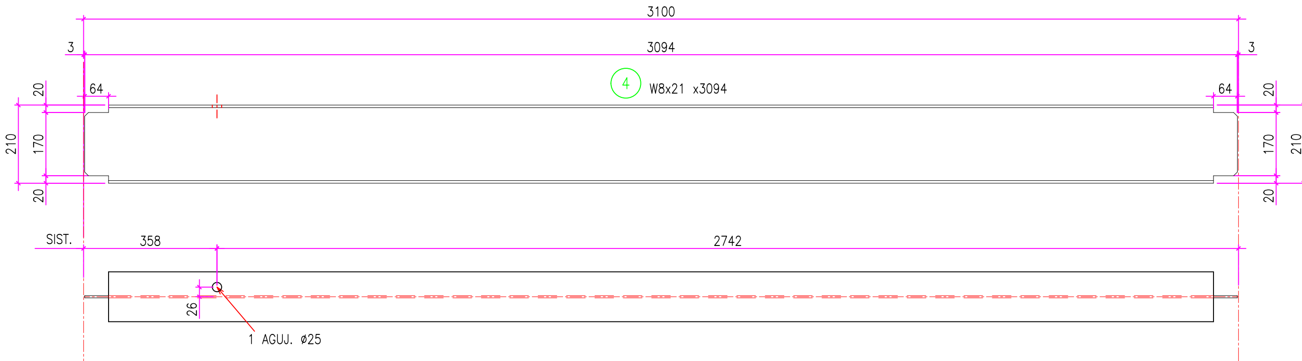
VIGA V5 CANT.: 3 ESC.: 1:10
