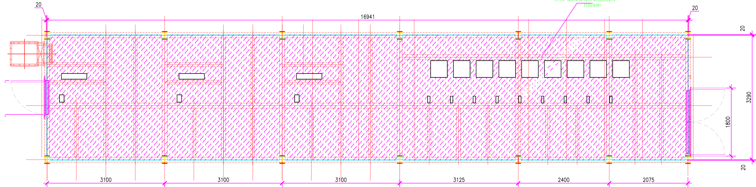
PLANTA CHAPA DE PISO PLATAFORMA PLT SEM-01 ESCALA 1:50
