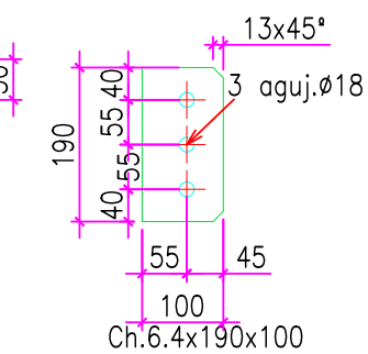
DET.POS 48 CANT.:13 ESC.1:10
