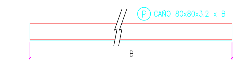
CORREAS LATERALES ESCALA 1:10
