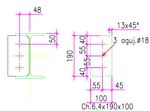
CORTE A
